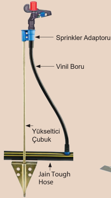
6025 SD U Turuncu ve Kırmızı Nozle için Montaj
